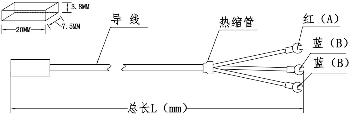
探头尺寸图
