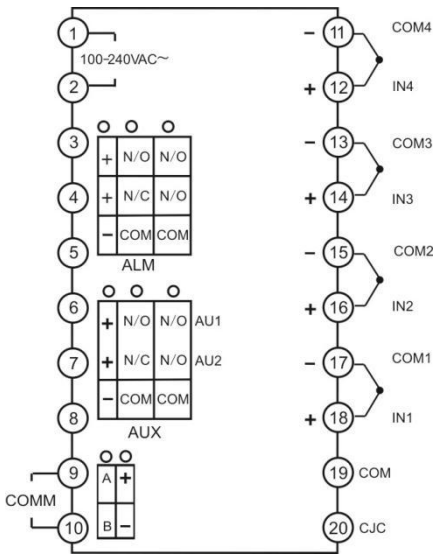
LD721/LD741 接线图如下：
