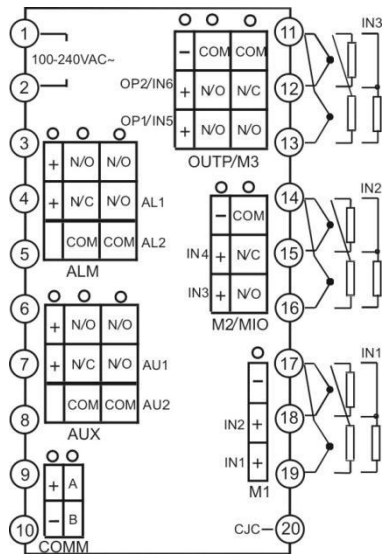
LD720/740/760 接线图如下：
